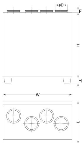
GS-VK 200 - 1900
